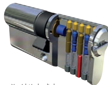
Vue éclatée du cylindre
